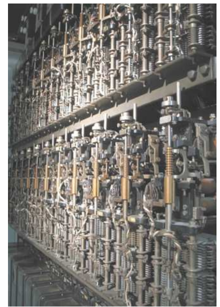
Hebendrehwählergestell vom Typ 22 der Firma Siemens
